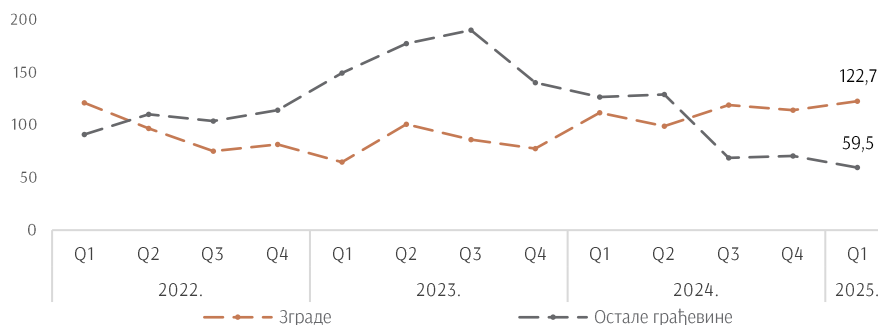
Вредност изведених грађевинских радова, према врсти грађевина, у АП Војводини, у сталним ценама (мг. индекси)
